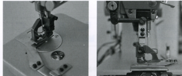
GC0388-GD 自动剪线上下复合送料缩缝缝纫机
